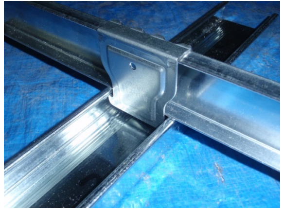
(d) 腹掛け（野縁受け腹側）
