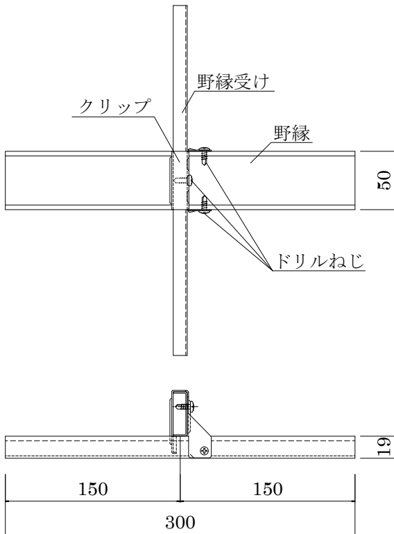
付図1.2 試験体の形状・寸法 (引張方向加力, 腹掛け)
