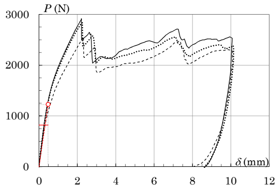
図1.1 荷重 P －変形 \delta 関係（引張方向加力，背掛け，評価方法1）
