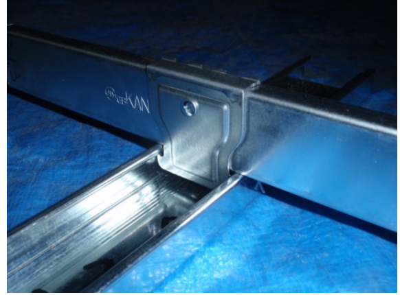
(b) 背掛け（野縁受け背側）
