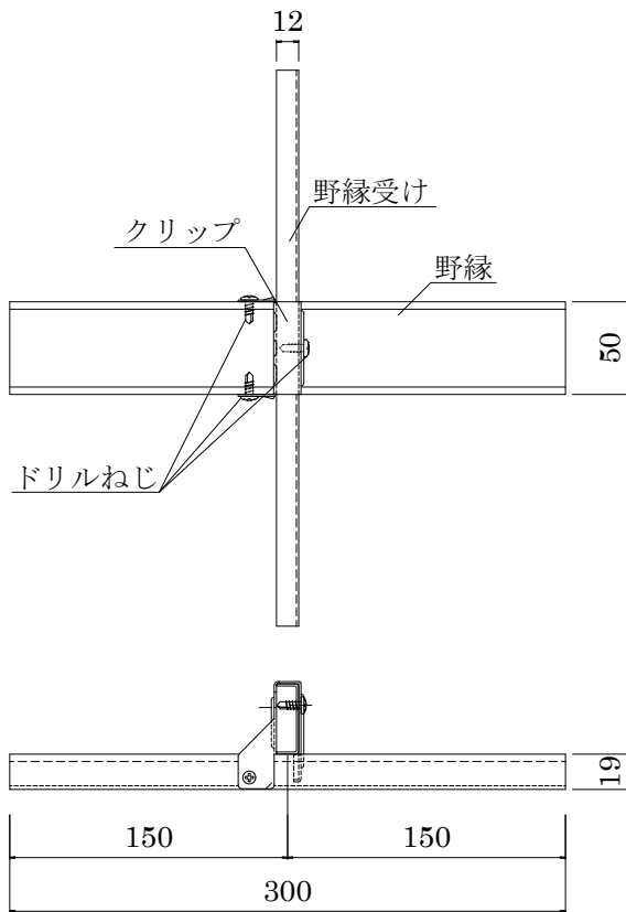
付図1.1 試験体の形状・寸法 (引張方向加力, 背掛け)
