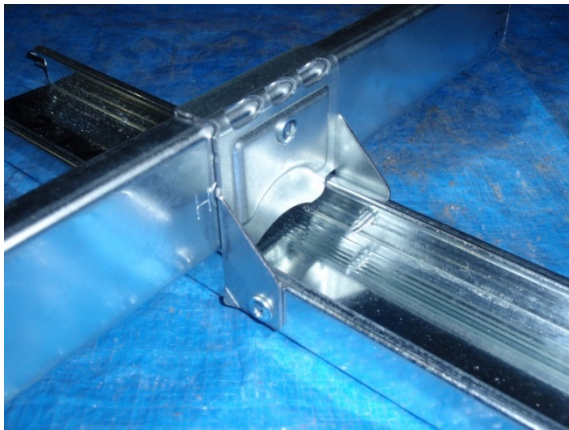
(c) 腹掛け（野縁受け背側）
