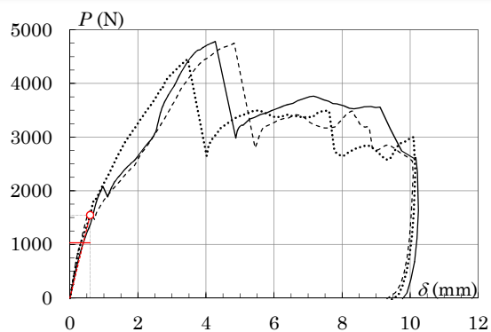
図1.2 荷重 P －変形 \delta 関係（引張方向加力，腹掛け，評価方法1）
