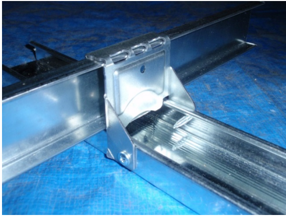
(a) 背掛け（野縁受け腹側）
