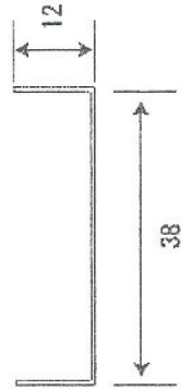
野縁受け
