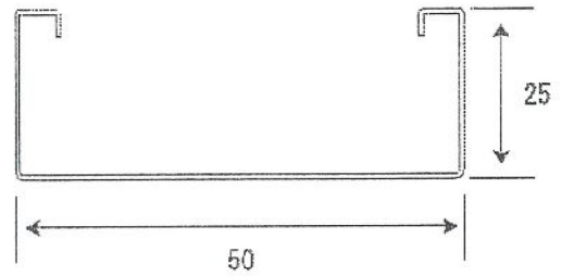
ダブル野縁
