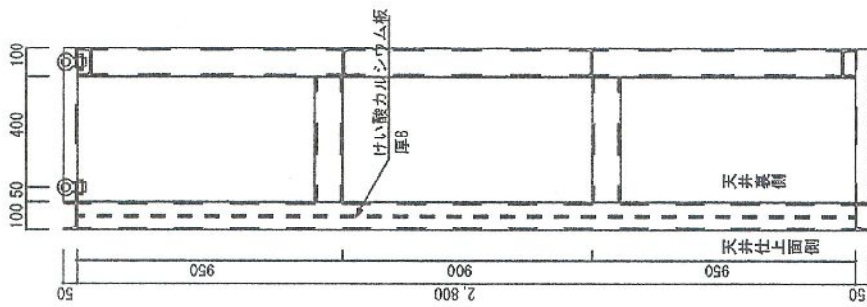
側面図
